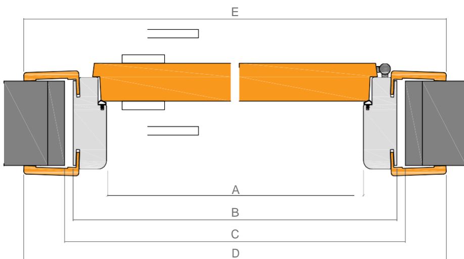
SEZIONE ORIZZONTALE
