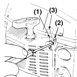
(1) Ago L ; (2) Ago H (3) Vite del minimo
