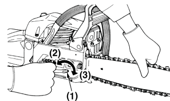
(1) Vis du tendeur ; (2) Desserrer ; (3) Serrer
