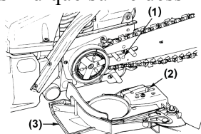
(1) Orifice ; (2) Ecrou de tension ; (3) Carter de chaîne
