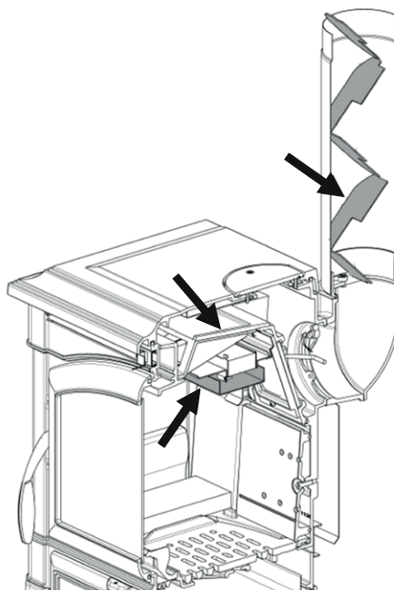
2 - DEFLETTORE FUMI
