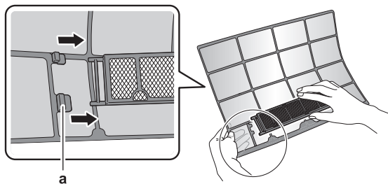
a Linguette
