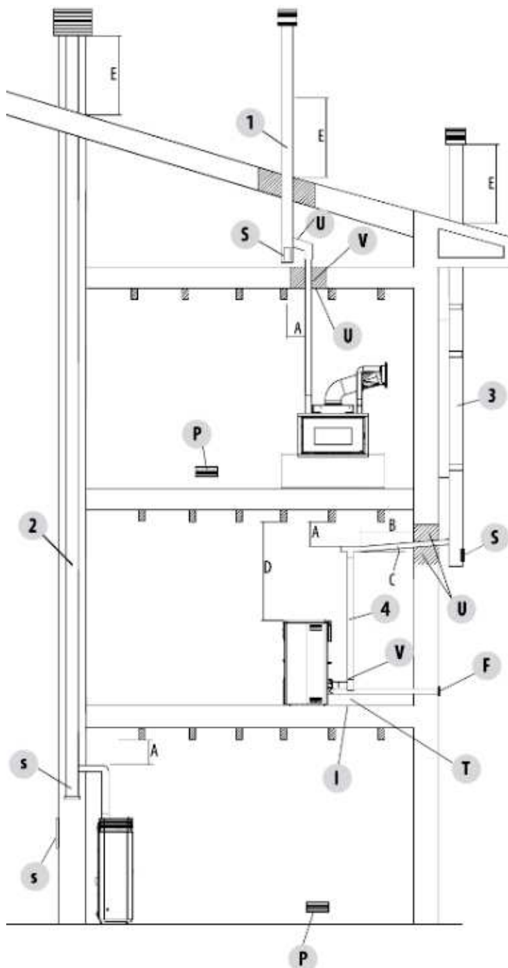
Fig. 13 - Canna fumaria
