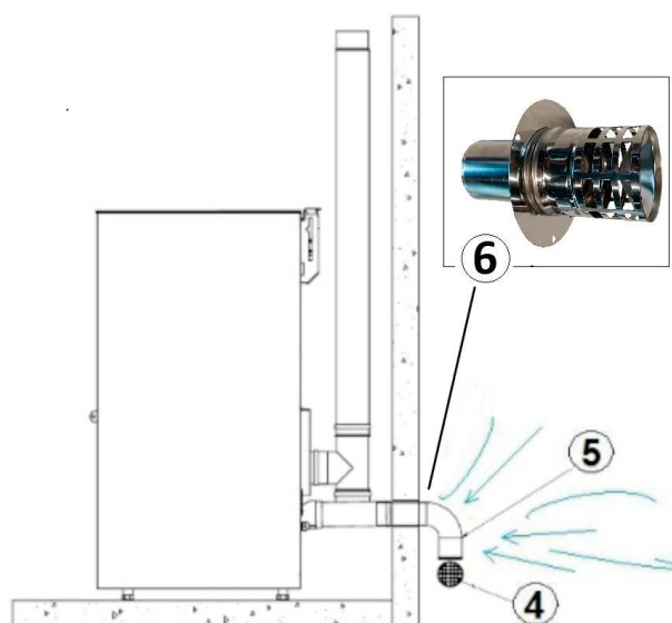
Fig. 8 - Presa d'aria per installazione a camera stagna
