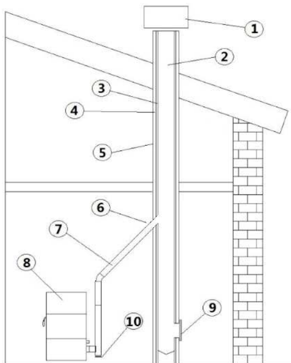
Fig. 2 - Componenti camino
