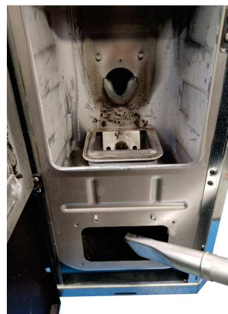
Fig. 83 - Aspirare cenere
