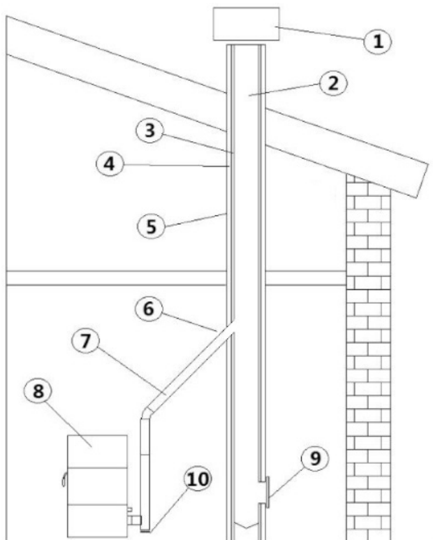
Fig. 2 - Componenti camino
