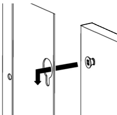
Fig. 25 - Dettaglio dell'aggancio
