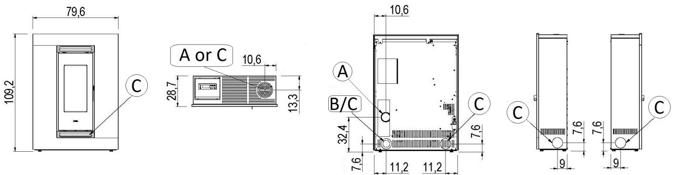
Fig. 13 - Luce Plus 9
