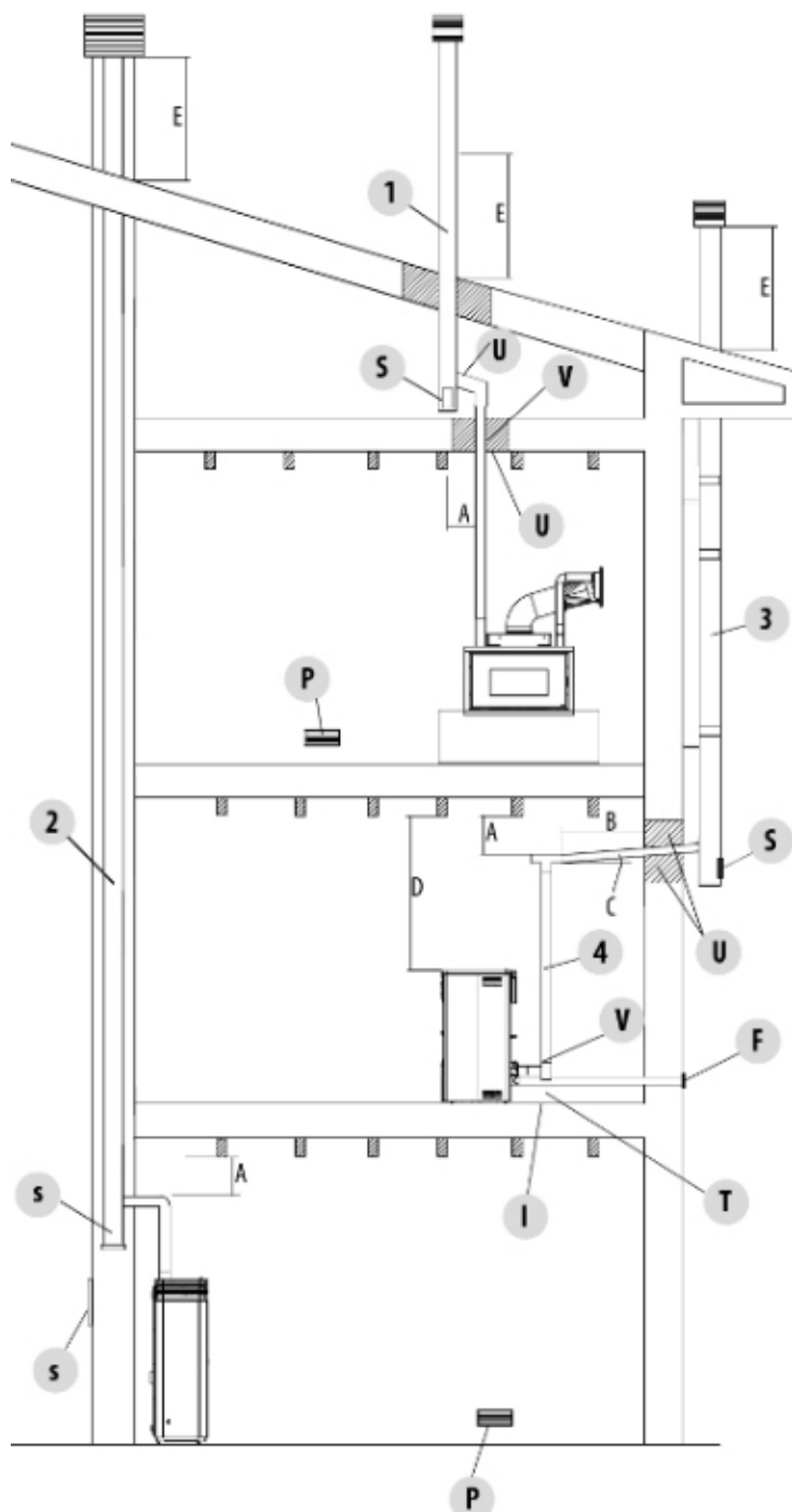
Fig. 11 - Canna fumaria
