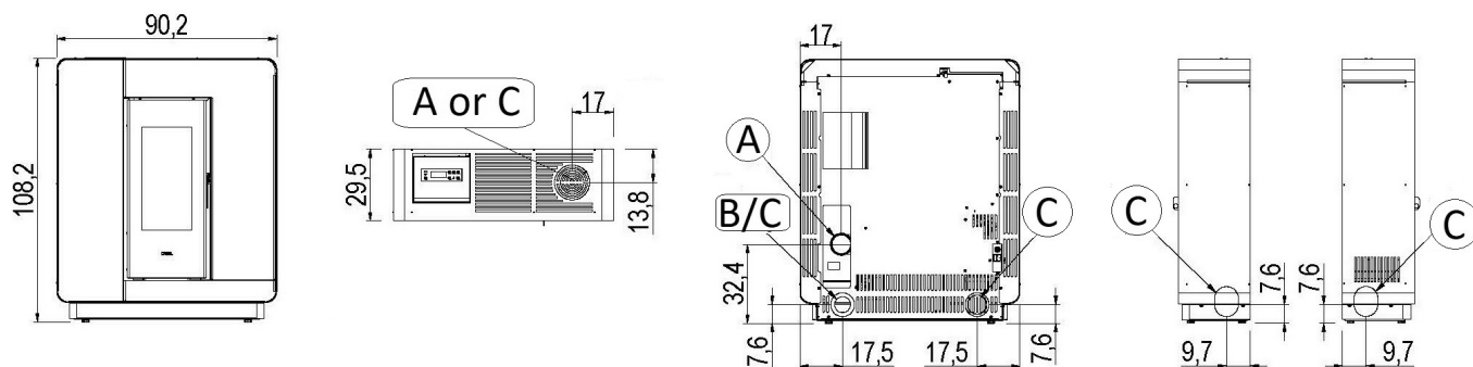
Fig. 15 - Elle Plus 9
