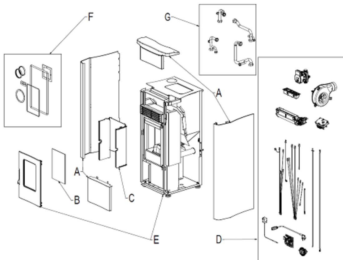
Fig. 1 - Esploso
