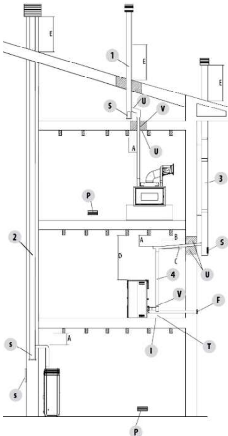
Fig. 11 - Canna fumaria
