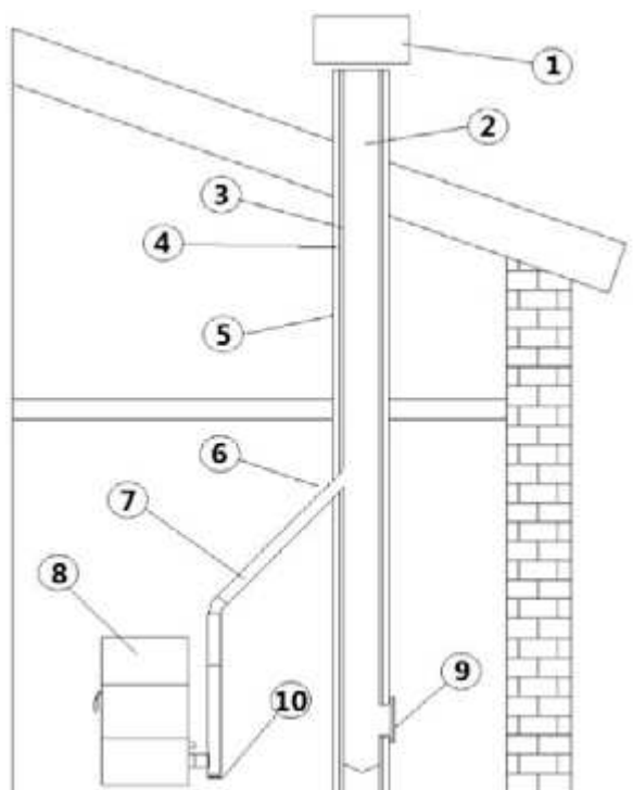
Fig. 2 - Componenti camino
