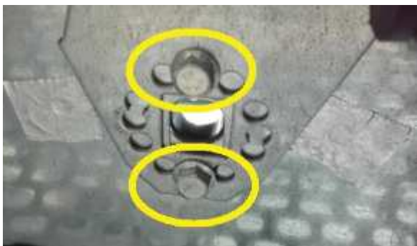
Fig. 74 - Rimozione viti
