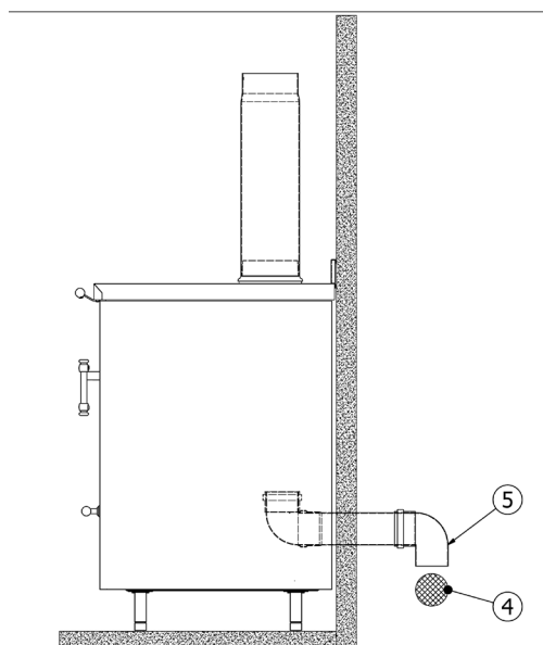
Fig. 7 - Installazione stagna
