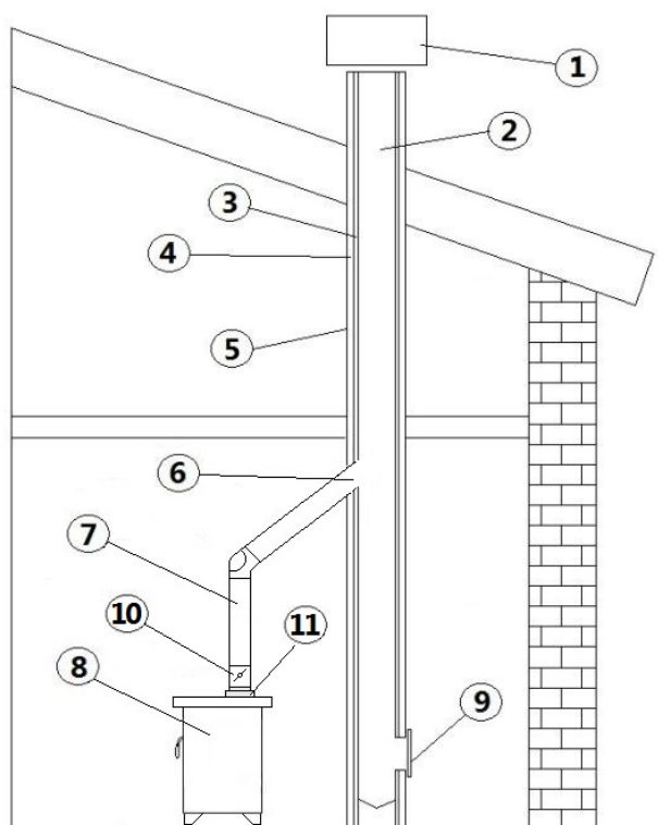
Fig. 2 - Componenti camino
