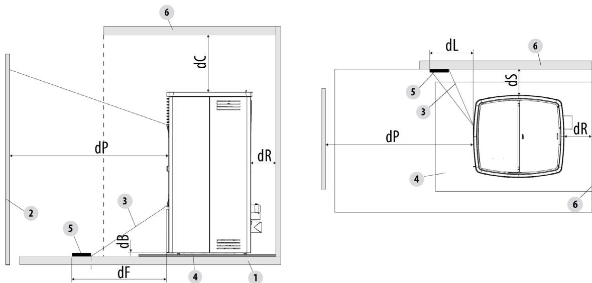
Fig. 13 - Distanze di sicurezza da materiale combustibile
