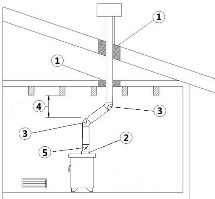
Fig. 8 - Esempio 1
