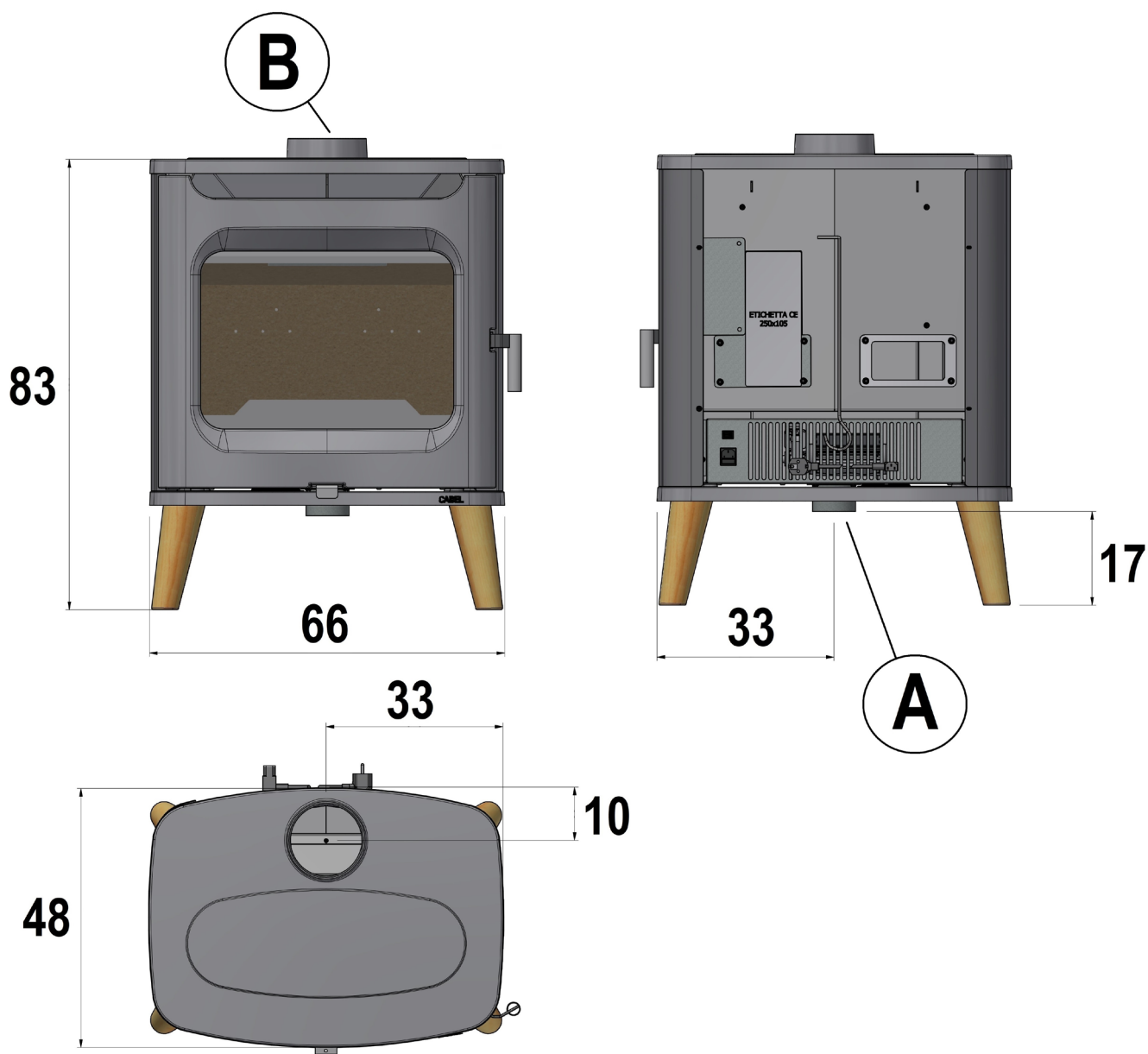
Fig. 12 - Dimensioni d'ingombro: FLOS Wood
