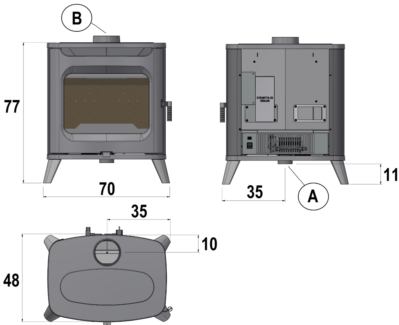
Fig. 11 - Dimensioni d'ingombro: HUBLOT Wood
