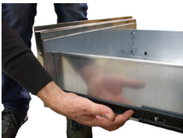
Fig. 26 - Sganciare guida
