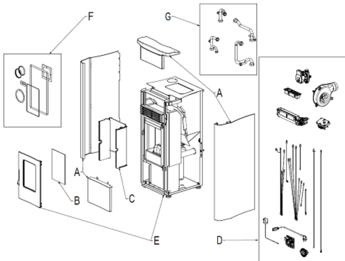
Fig. 2 - Esploso
