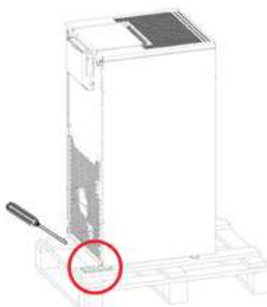
Fig. 1 - Rimozione staffe
