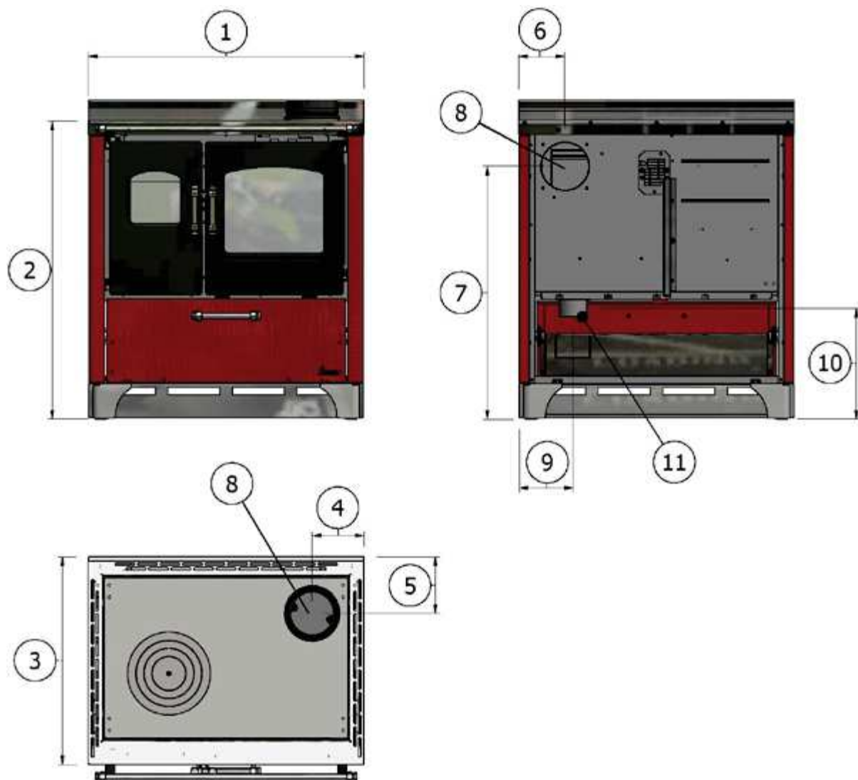
Fig. 14 - Dimensioni d'ingombro: SMART 80
