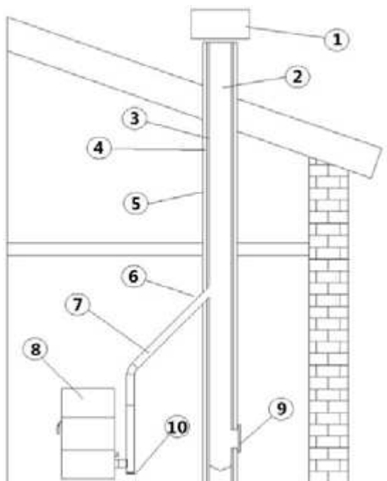
Fig. 2 - Componenti camino
