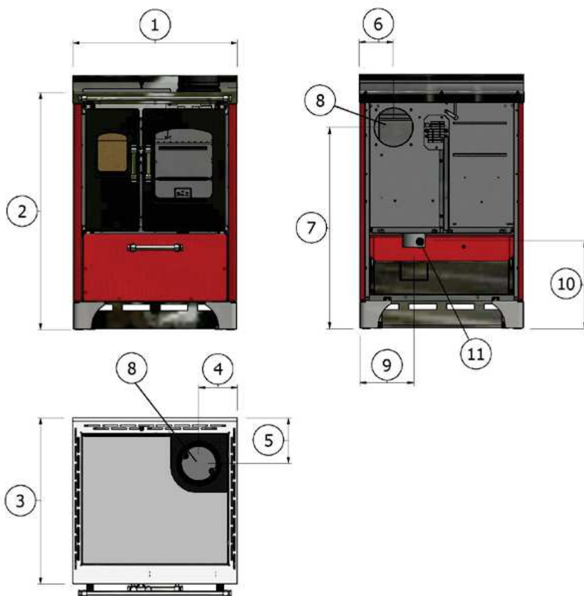
Fig. 13 - Dimensioni d'ingombro: SMART 60
