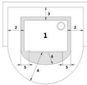
Fig. 15 - Installazione generica
