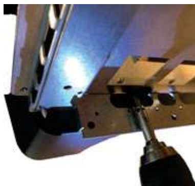
Fig. 43 - Montaggio piedini 2
