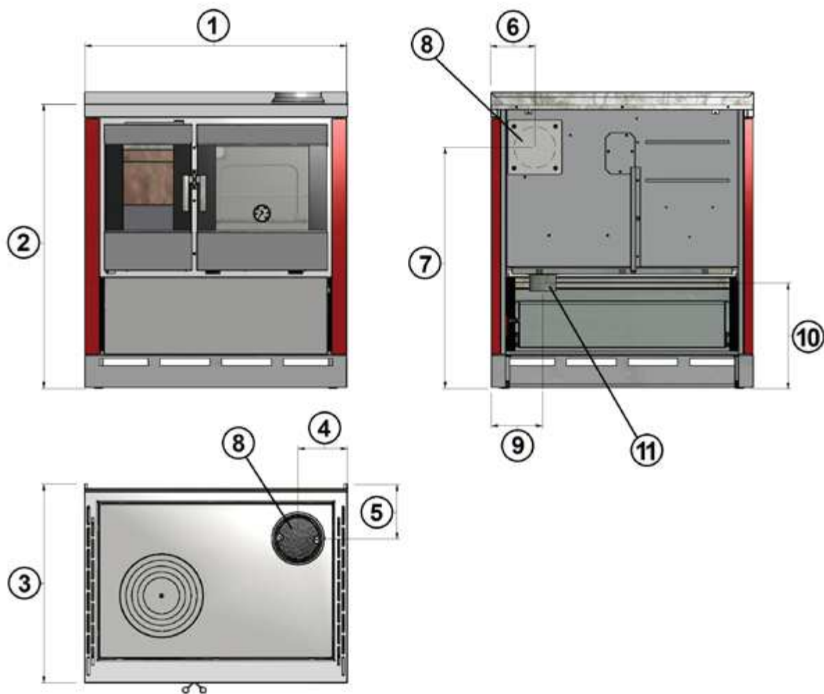
Fig. 12 - Dimensioni d'ingombro: Kook 80 - Kook 90
