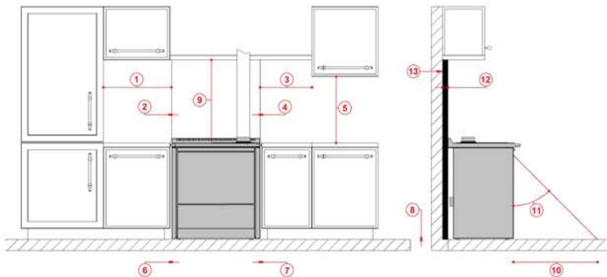
Fig. 16 - Installazione ad incasso
