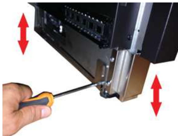
Fig. 18 - Regolazione profilo zoccolo: Kook 60
