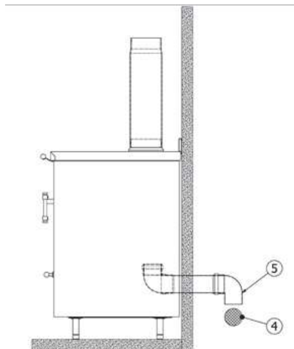
Fig. 7 - Installazione stagna
