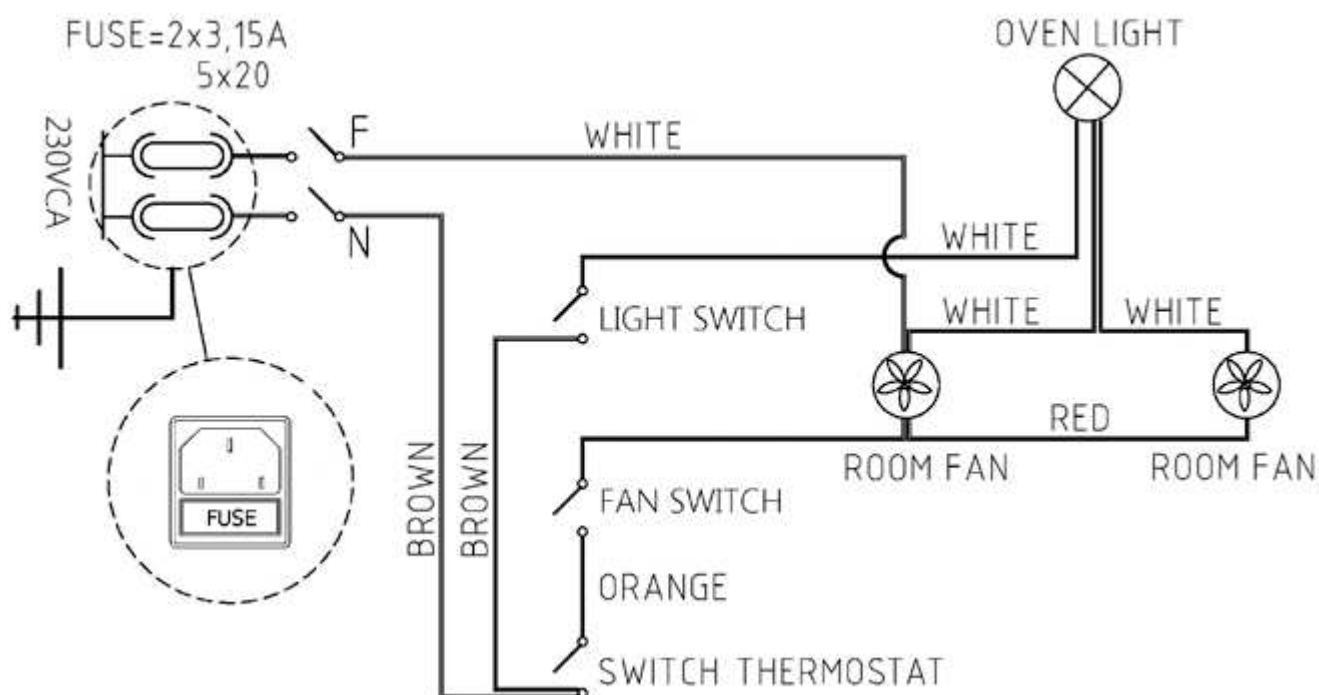
Fig. 76 - Schema elettrico
