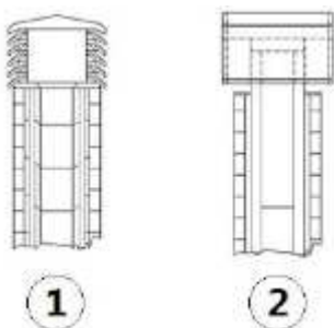
Fig. 4 - Comignoli antivento
