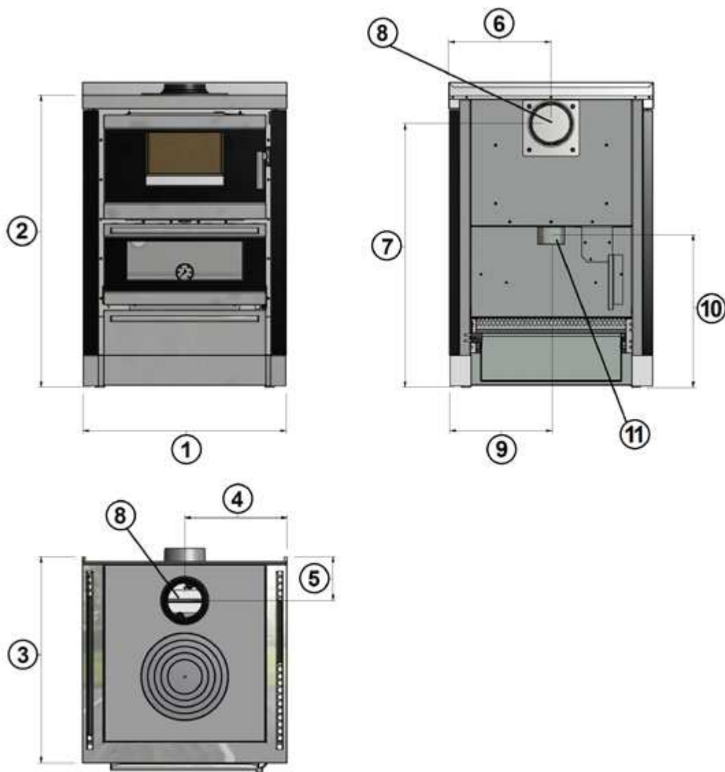
Fig. 11 - Dimensioni d'ingombro: Kook 60
