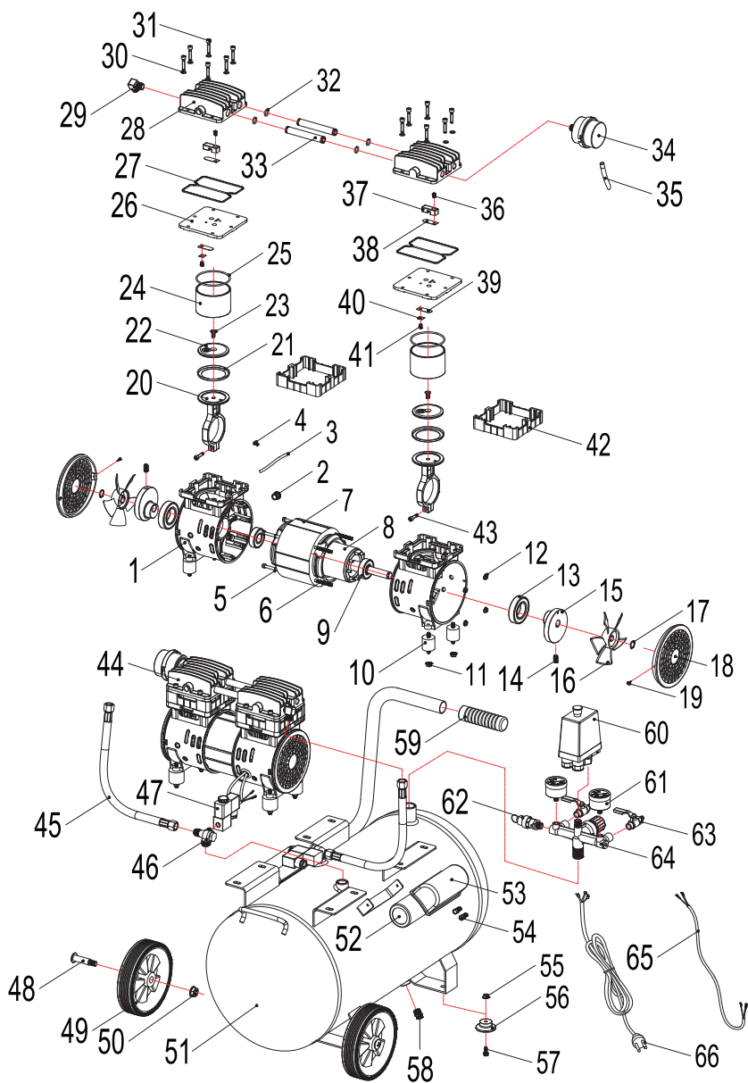
Compressore PH050S2
