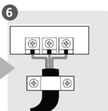
6. Bedrading aansluiten (niet van toepassing voor sommige plaatsen in Noord-Amerika)
