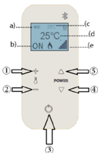
Fig. 29 - Telecomando con termostato
