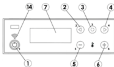
Fig. 7 - Pannello di controllo (wi-fi)
