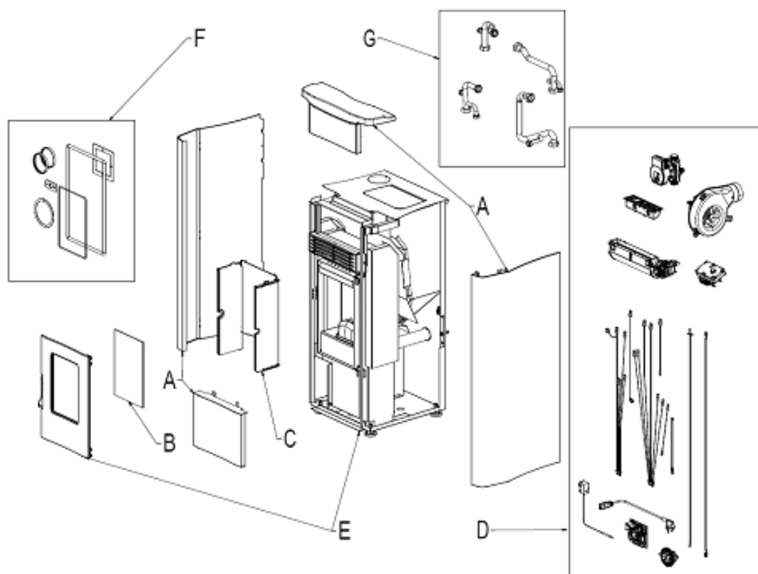
Fig. 1 - Esploso
