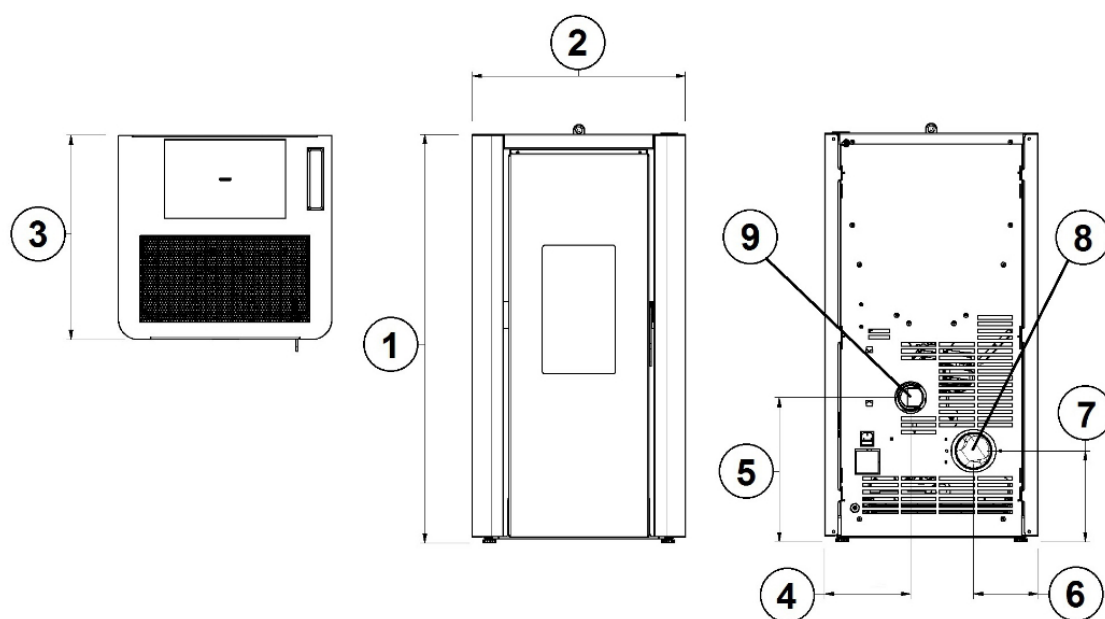
Fig. 23 - Dimensioni generali: INDIGO 7
