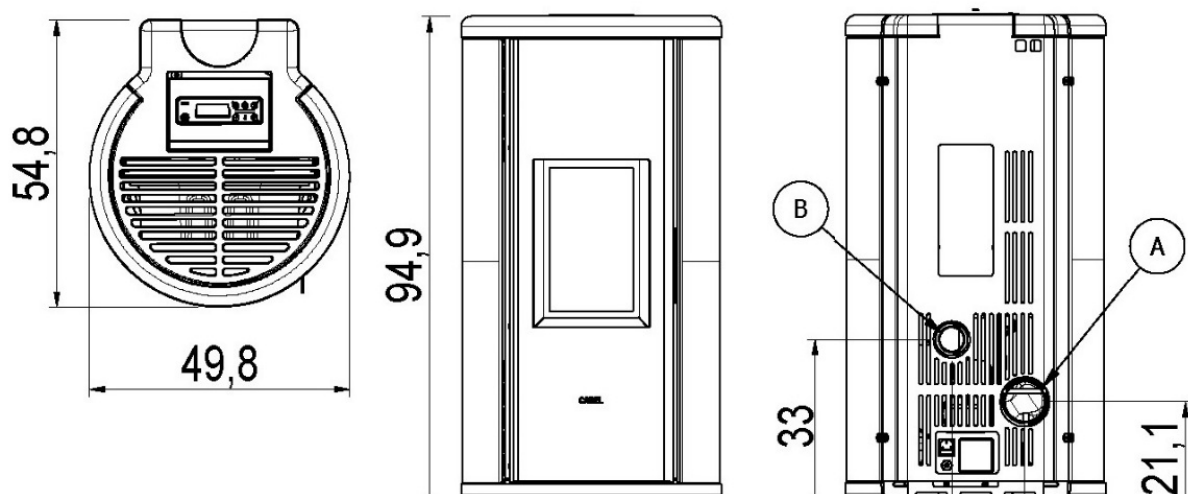
Fig. 17 - Dimensioni generali: SOUND SPS - 7PS
