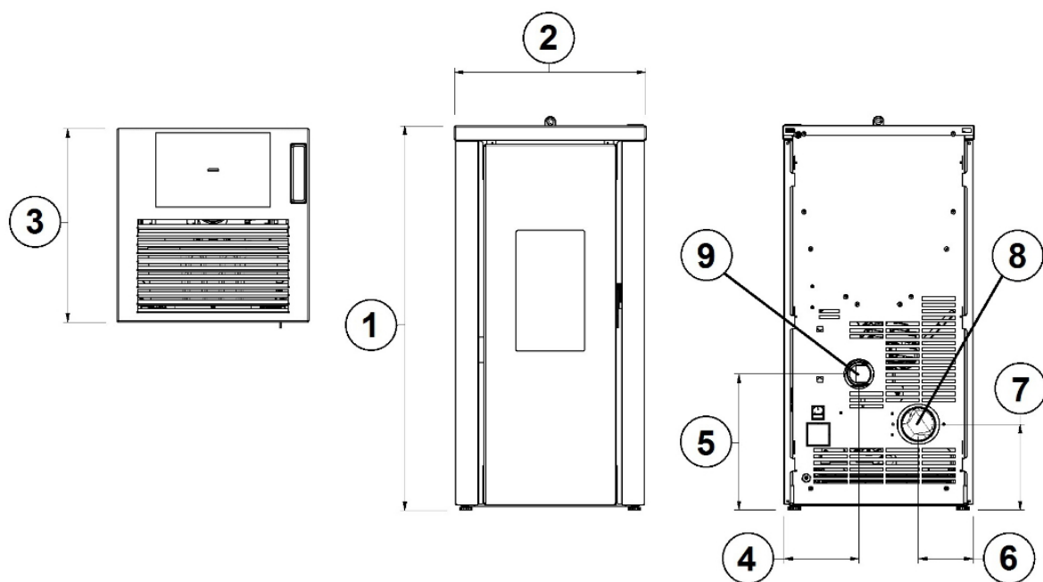
Fig. 22 - Dimensioni generali: VERA 7
