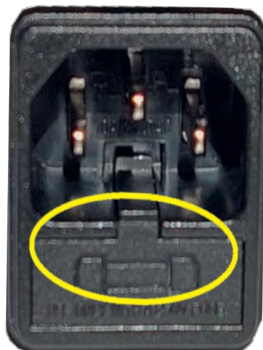
Fig. 78 - Sportellino con i fusibili da rimuovere
