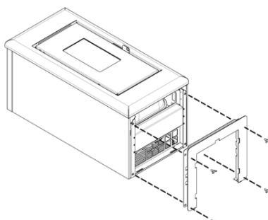
Fig. 46 - Montaggio piedistallo
