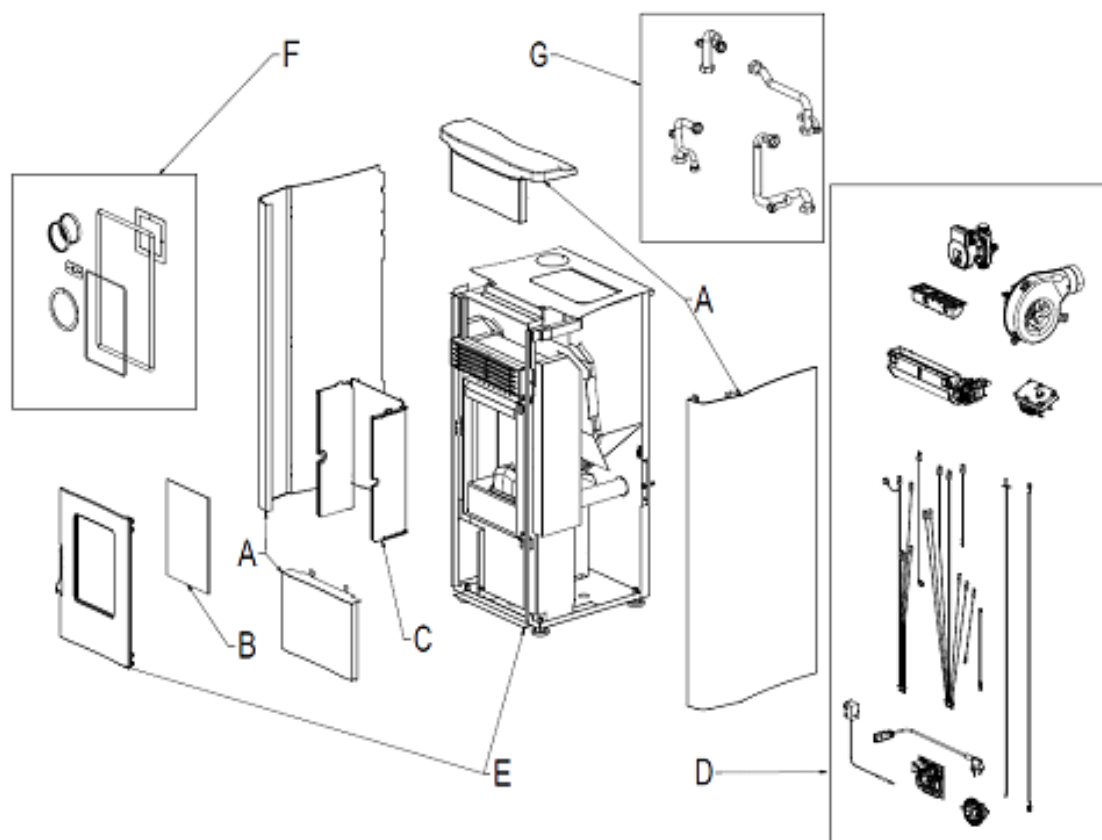
Fig. 1 - Esploso
