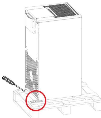
Fig. 1 - Rimozione staffe
