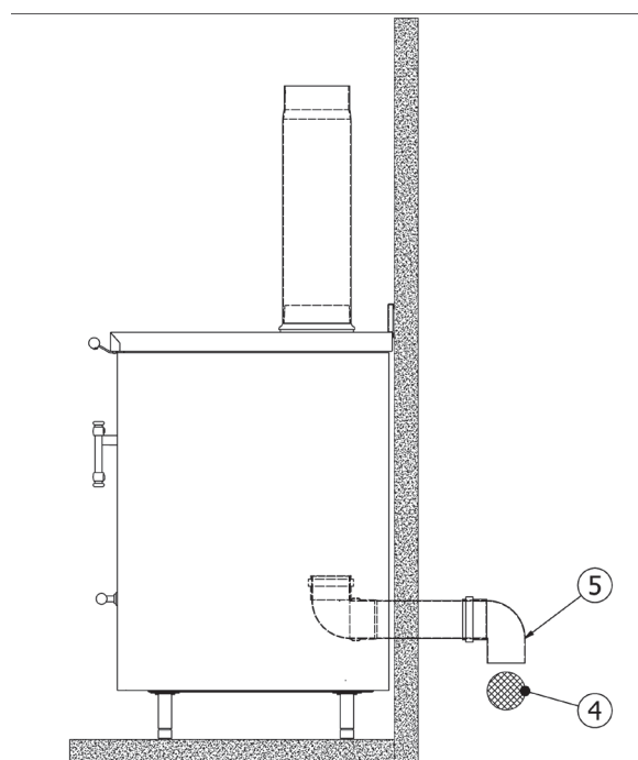
Fig. 7 - Installazione stagna
