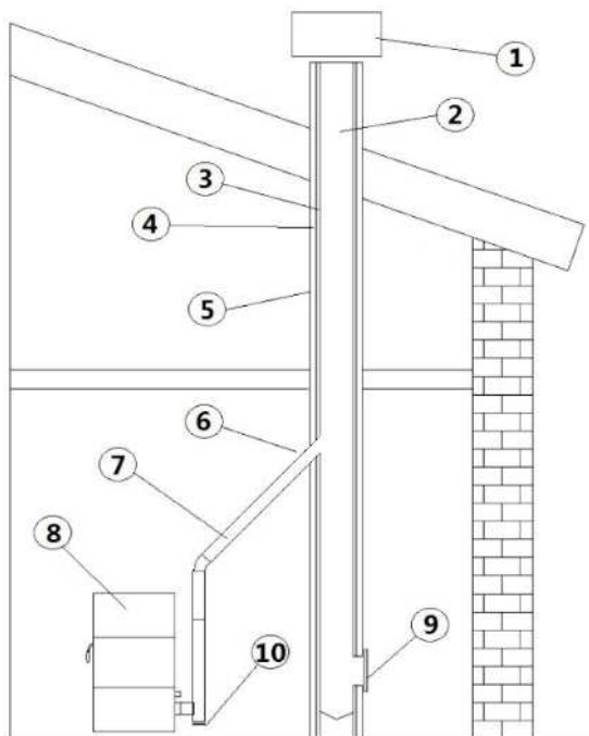
Fig. 2 - Componenti camino
