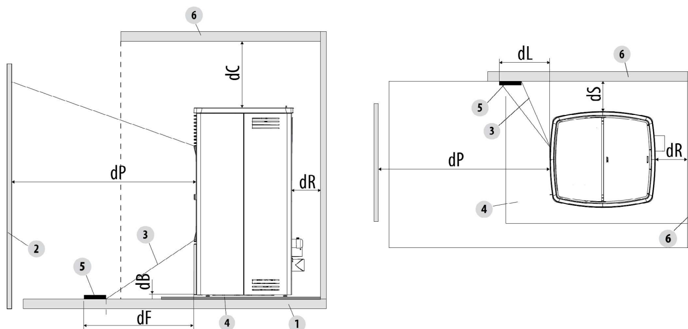
Fig. 11 - Distanze di sicurezza da materiale combustibile
