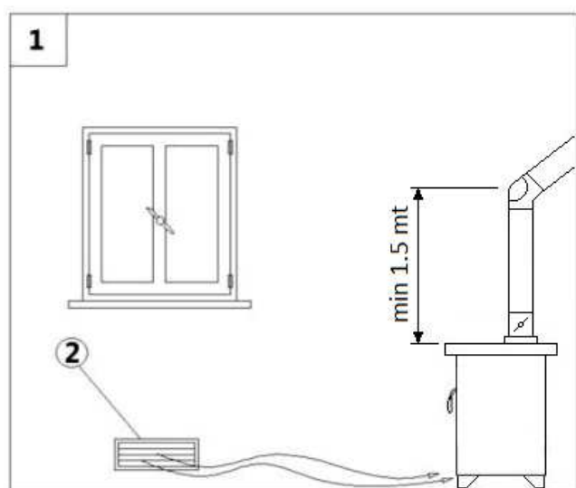
Fig. 6 - Afflusso d'aria diretta
