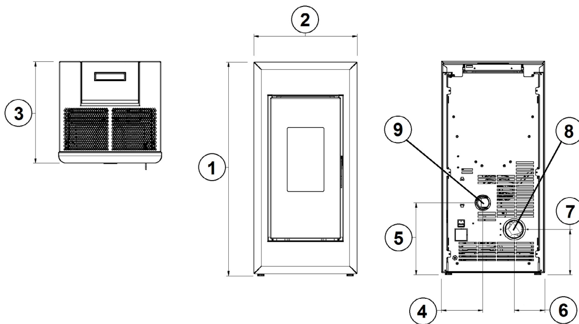
Fig. 20 - Dimensioni generali: ONE7 - BEAM 7 - ACCENT K7
