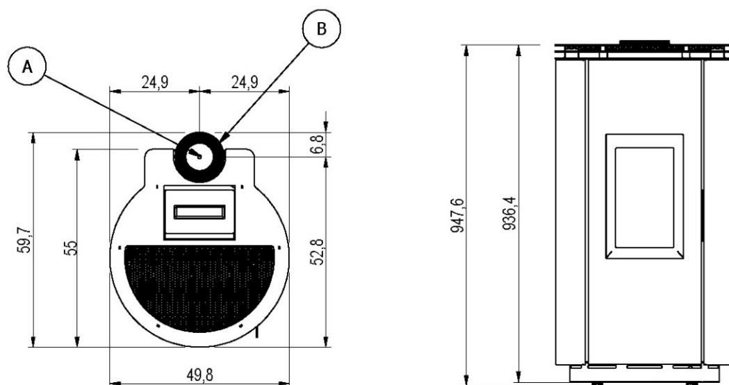
Fig. 19 - Dimensioni generali : FLOYD 5-7 - LORD 7
