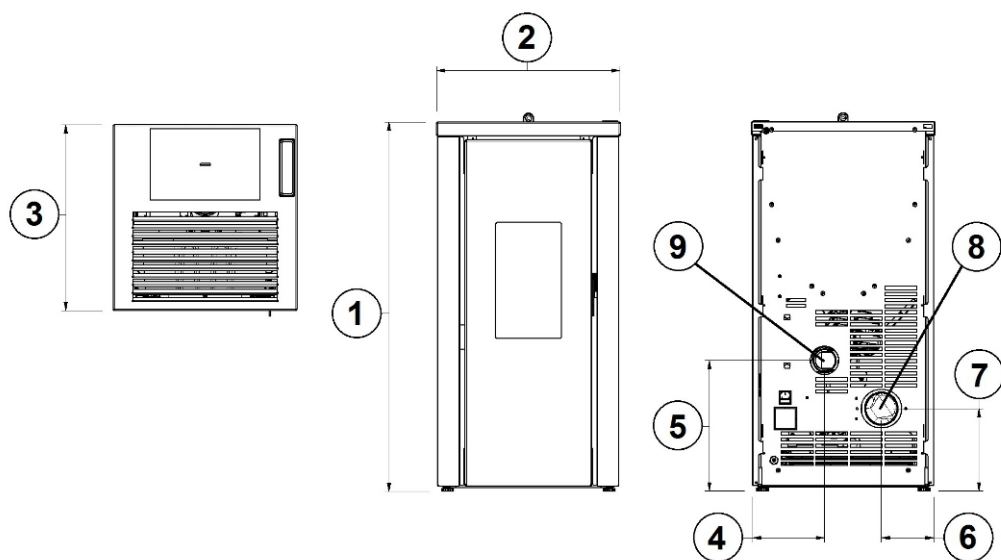
Fig. 23 - Dimensioni generali: VERA 7
