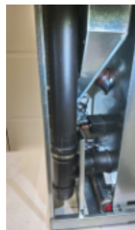
Fig. 54 - Raccordo "T"
