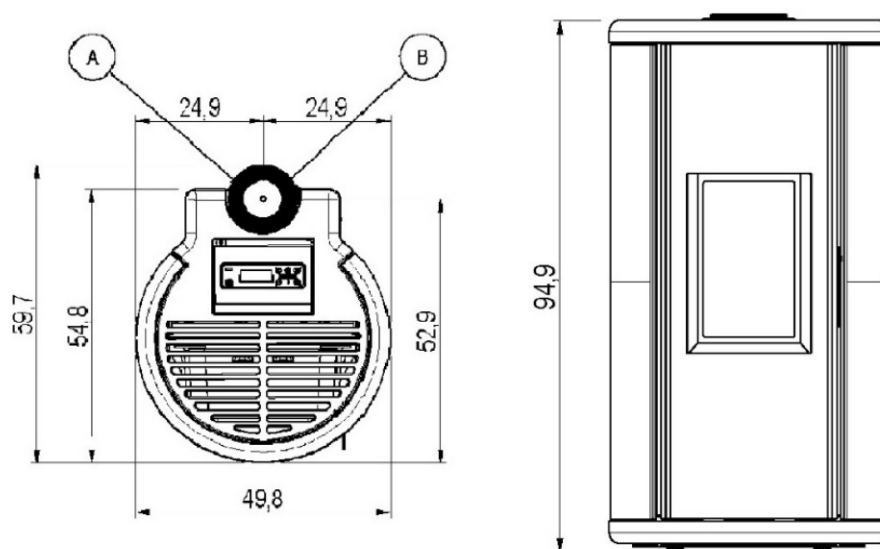
Fig. 16 - Dimensioni generali: SOUND SUP-Twin - 7UP-Twin
