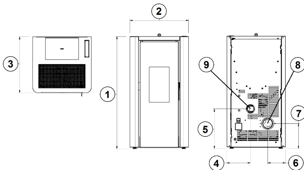
Fig. 24 - Dimensioni generali: INDIGO 7
