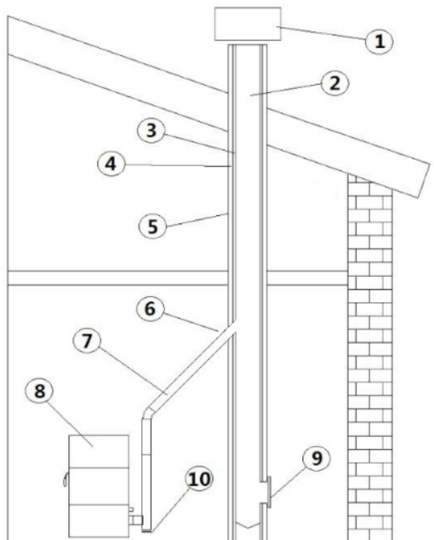
Fig. 2 - Componenti camino
