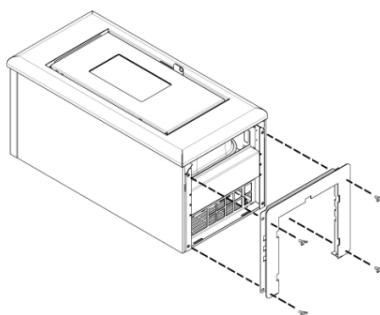
Fig. 48 - Montaggio piedistallo
