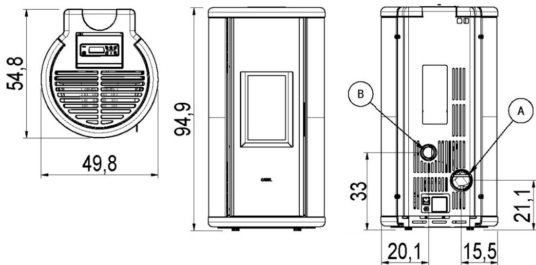
Fig. 17 - Dimensioni generali: SOUND 5PS - 7PS
