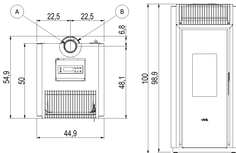
Fig. 22 - Dimensioni generali: BOLD 7 UP TWIN
