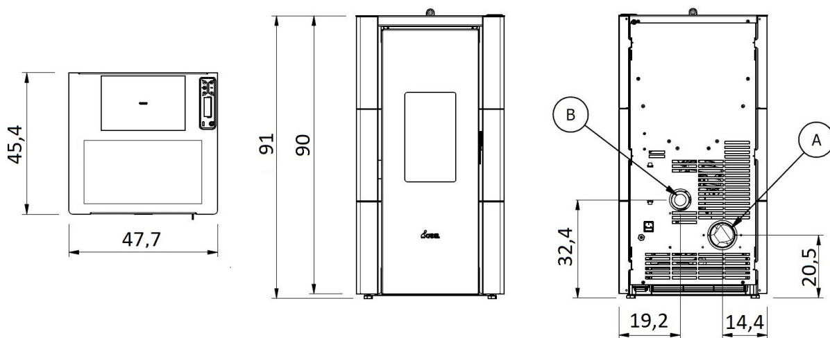
Fig. 14 - Dimensioni generali: CRISTAL 7 - LEE 7
