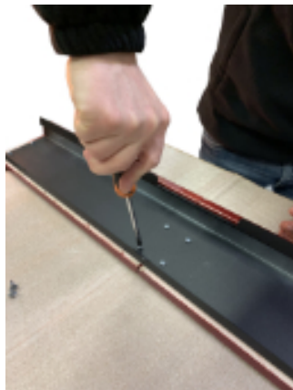
Fig. 45 - Montaggio maioliche
