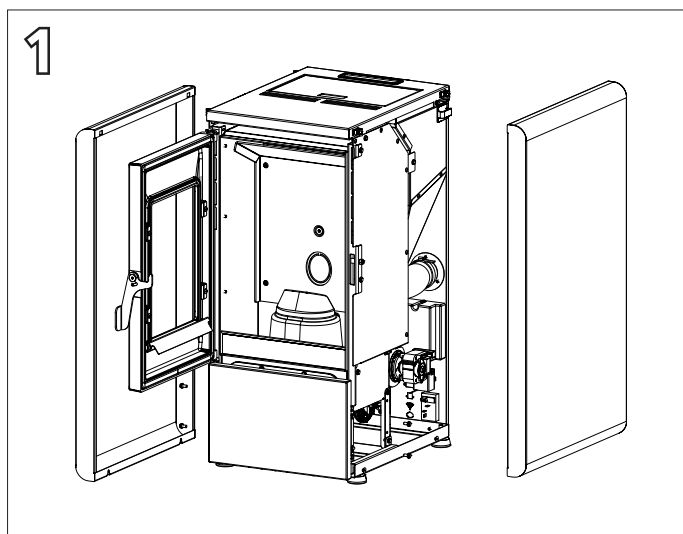
Rimuovere i fianchi.
