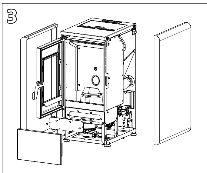
Rimuovere le viti e la piastra di ispezione.
