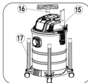
Assemblare gli accessori per la cenere
