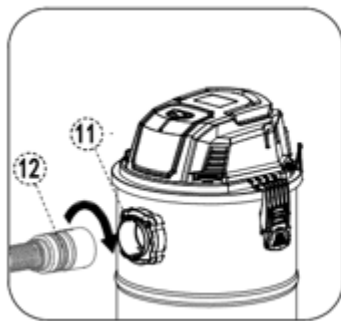
Inserire il flessibile
