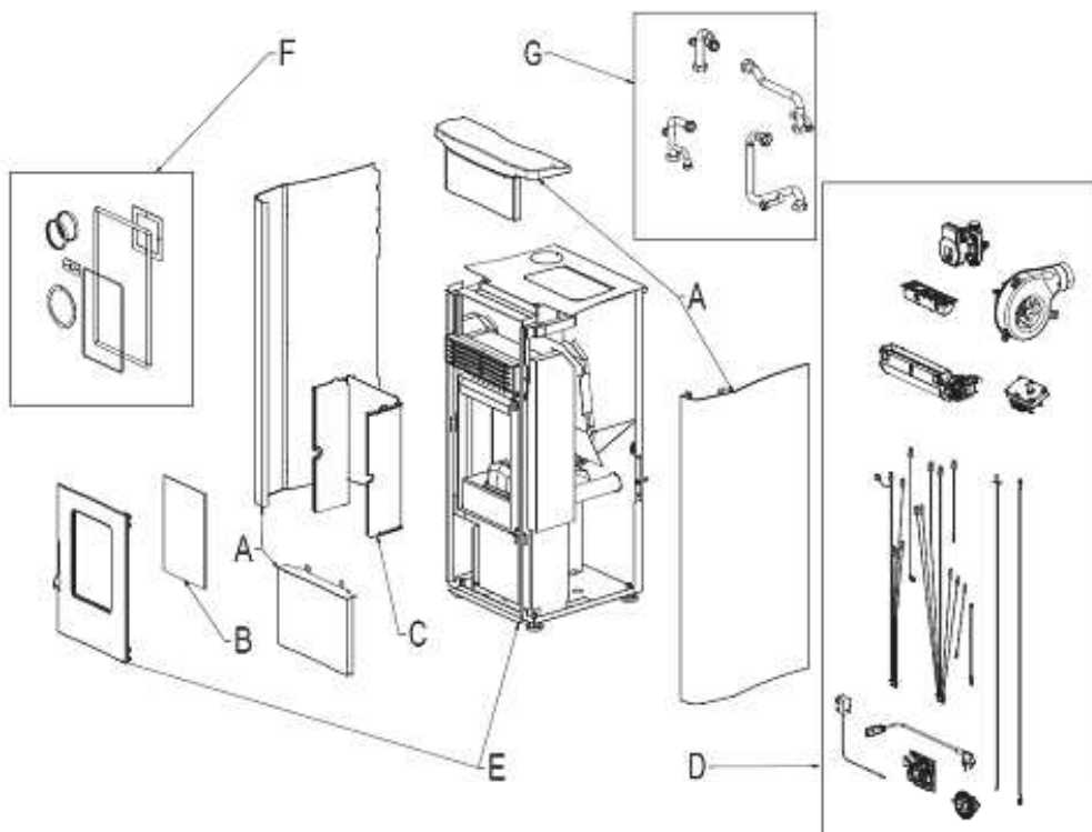
Fig. 1 - Esploso
