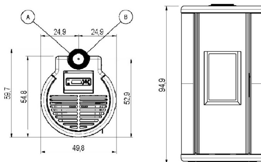
Fig. 17 - Dimensioni generali: SOUND SUP - 7UP
