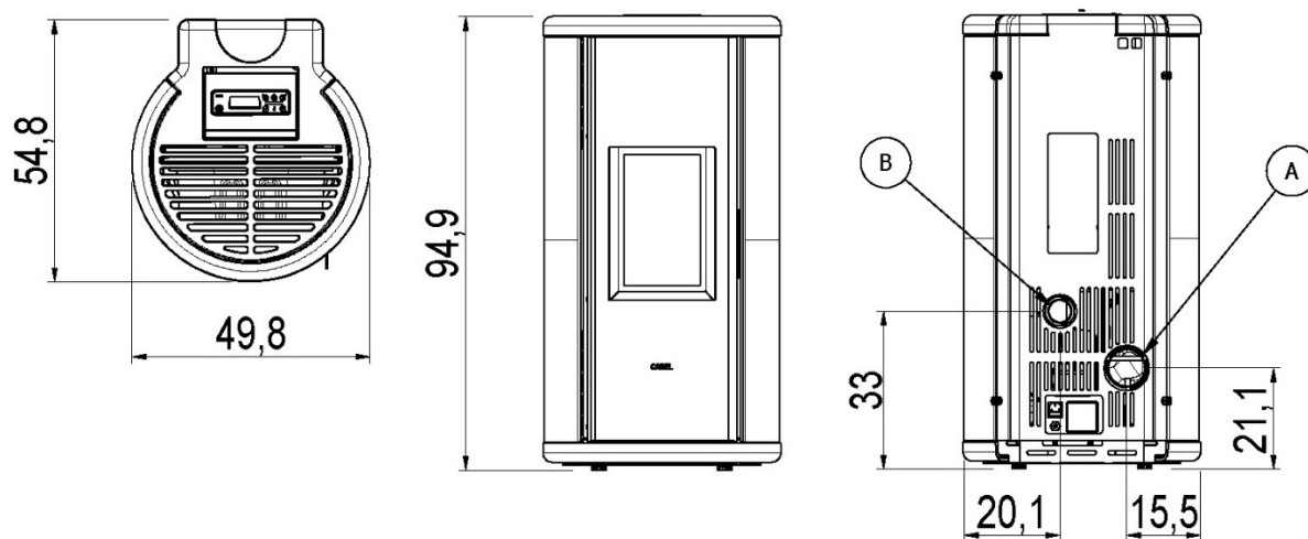
Fig. 18 - Dimensioni generali: SOUND 5PS - 7PS
