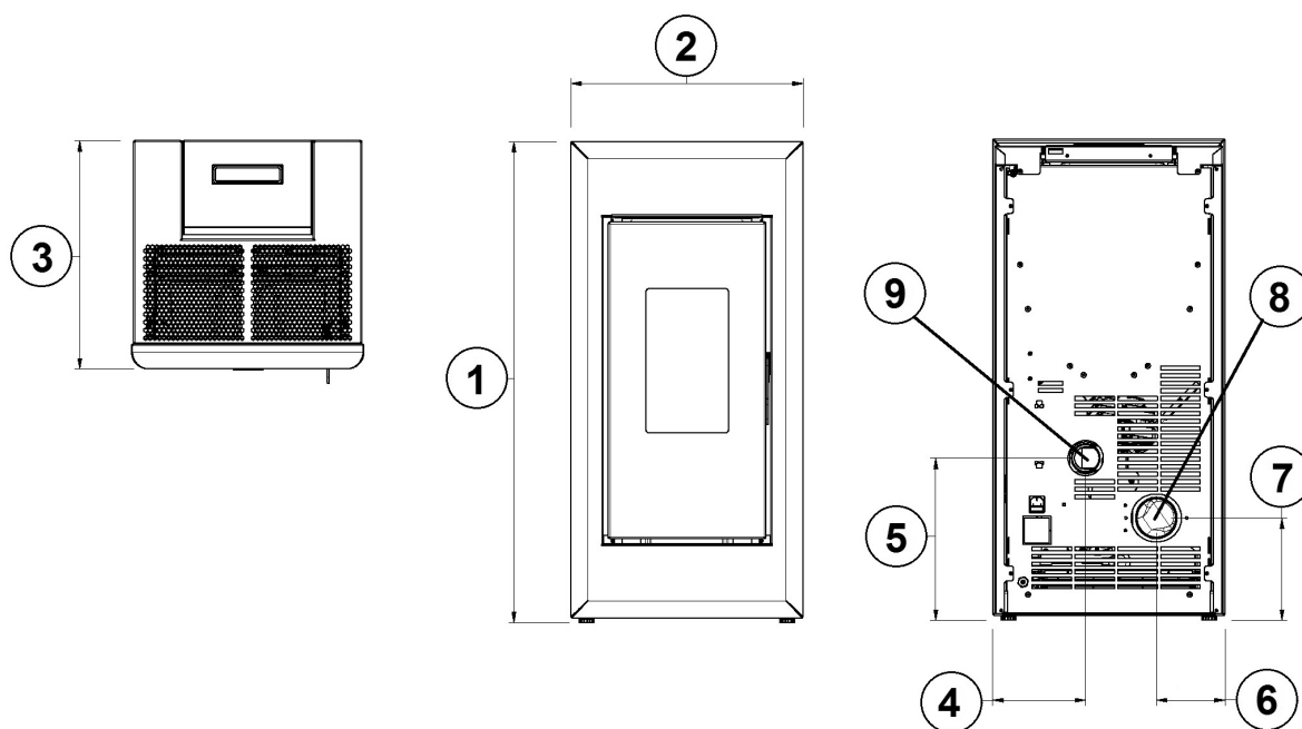
Fig. 21 - Dimensioni generali: ONE/BEAM AIRTIGHT
