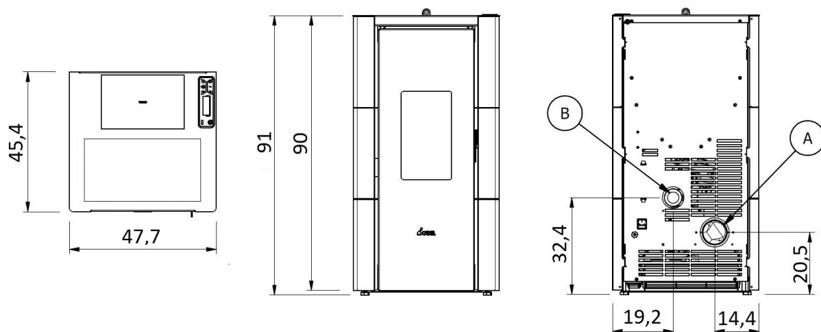
Fig. 15 - Dimensioni generali: CRISTAL - CRISTAL 7.0
