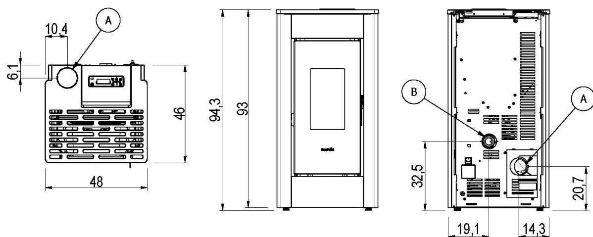
Fig. 16 - Dimensioni generali: SHARP AIRTIGHT - LEE AIRTIGHT
