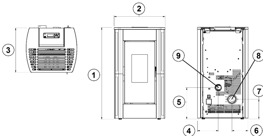
Fig. 14 - Dimensioni generali: PERLA 7 - 7.0
