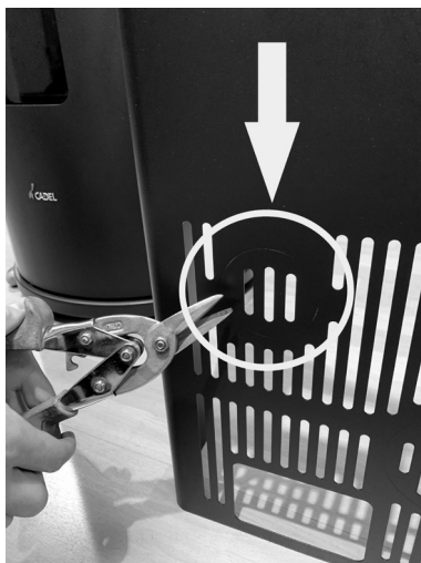
Fig. 54 - Rompere anello
