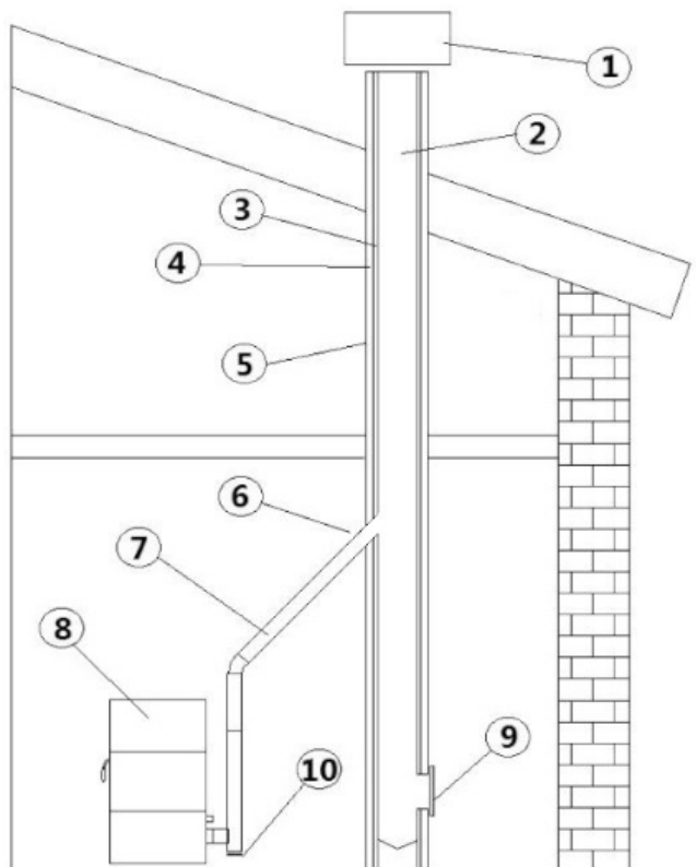
Fig. 2 - Componenti camino
