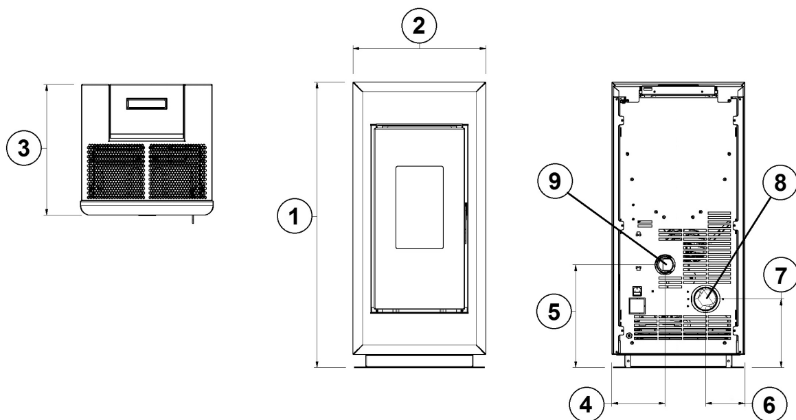
Fig. 22 - Dimensioni generali: ACCENT AIRTIGHT
