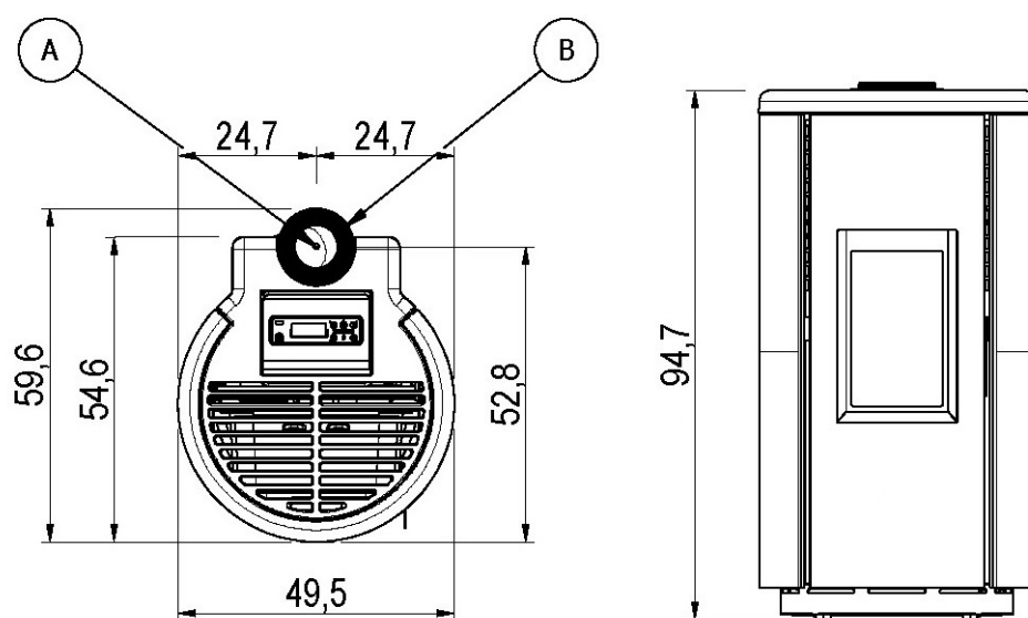
Fig. 19 - Dimensioni generali: CHROME 5-7 AIRTIGHT - ROUND 5-7 AIRTIGHT
