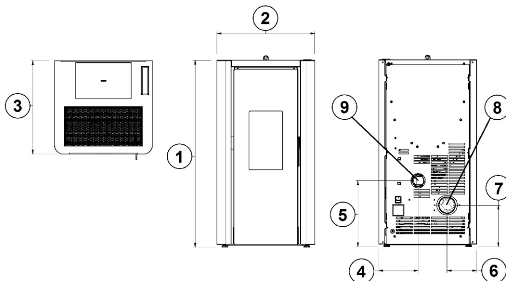
Fig. 24 - Dimensioni generali: INDIGO EVO 7
