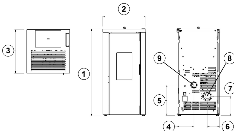
Fig. 12 - Dimensioni generali: LORD 7 - 7.0
