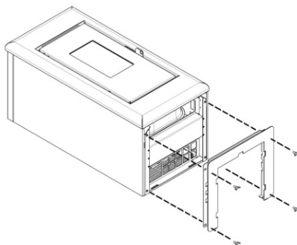
Fig. 45 - Montaggio piedistallo
