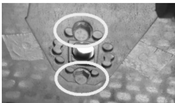
Fig. 78 - Rimozione viti
