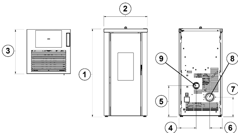
Fig. 23 - Dimensioni generali: VERA 7 - 7.0
